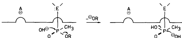
Schema 4. Hydroxy-Austausch
